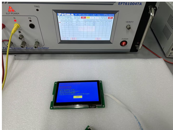
图 4-3 EFT 测试图
